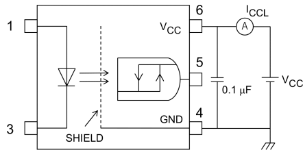
図 12.1.3 I_{CCL} 測定回路
