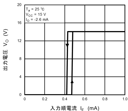
図 12.2.13 V_O - I_F
