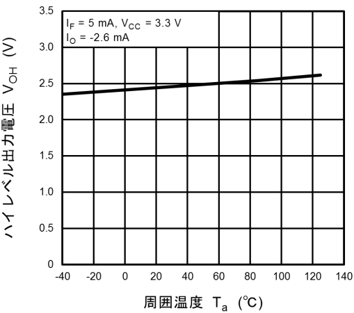
図 12.2.4 V_{OH} - T_a
