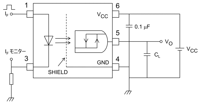
図 12.1.8 伝搬遅延時間測定回路, 波形
