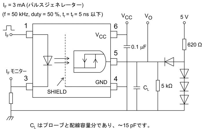
図 12.1.7 伝搬遅延時間測定回路, 波形
