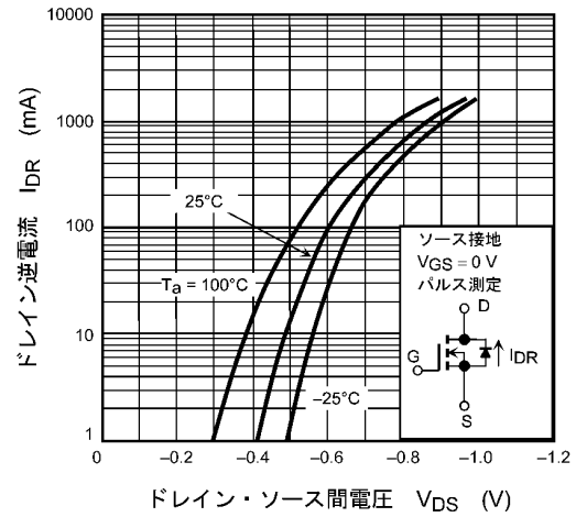
図 7.8 I_{DR} - V_{DS}
