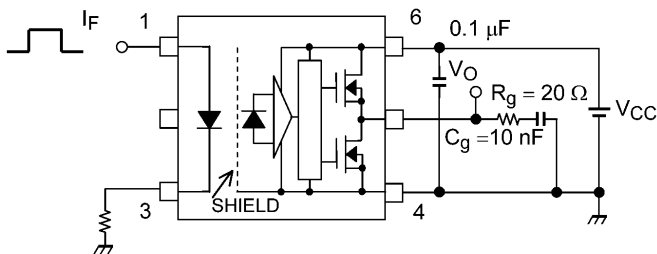
図 13.1.8 伝搬遅延時間測定回路, 波形
