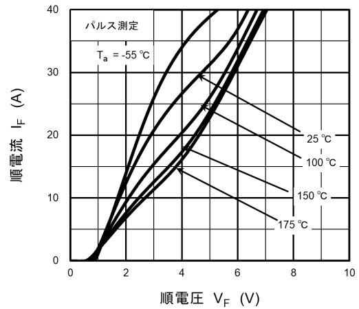
図 9.2 I_F - V_F
