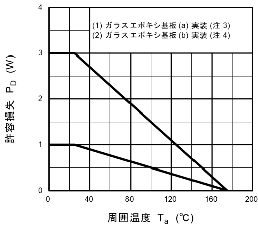
図 8.15 P_D - T_a (最大値 (保証値))
