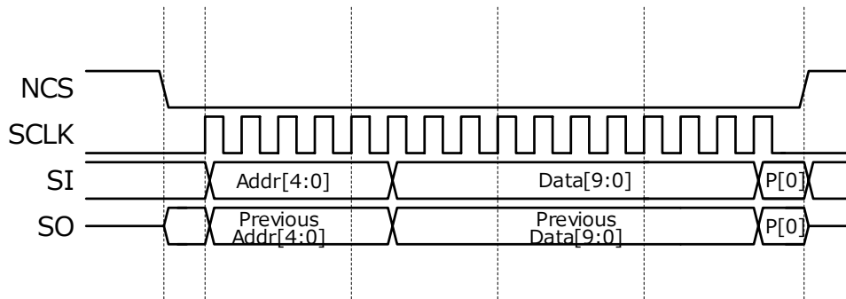
Fig. 7.8.1.1 Frame Format
