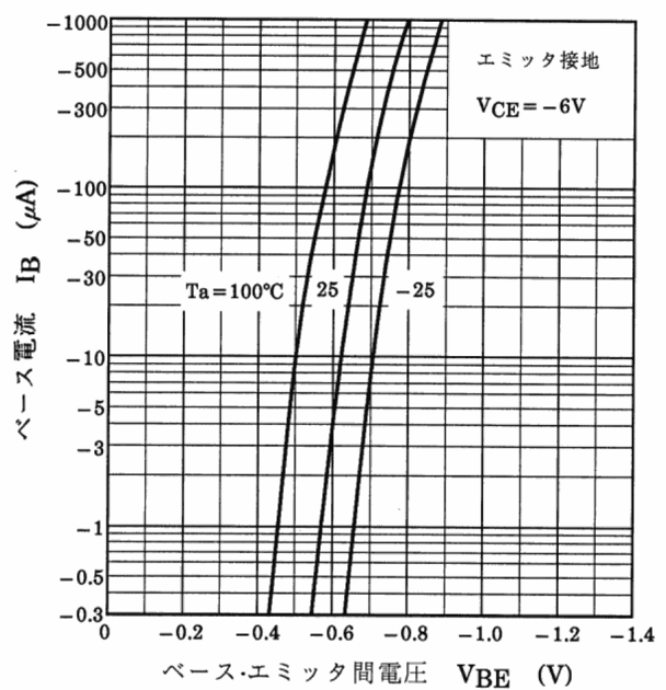
図 13.6 I_B - V_{BE}
