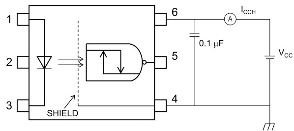
Fig. 13.1.4 I_{CCH} Test Circuit
