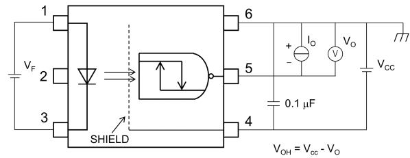
Fig. 13.1.2 V_{OH} Test Circuit
