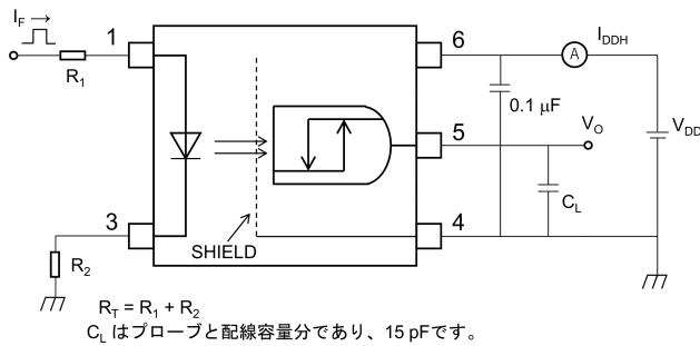
図 13.1.5 伝搬遅延時間測定回路, 波形
