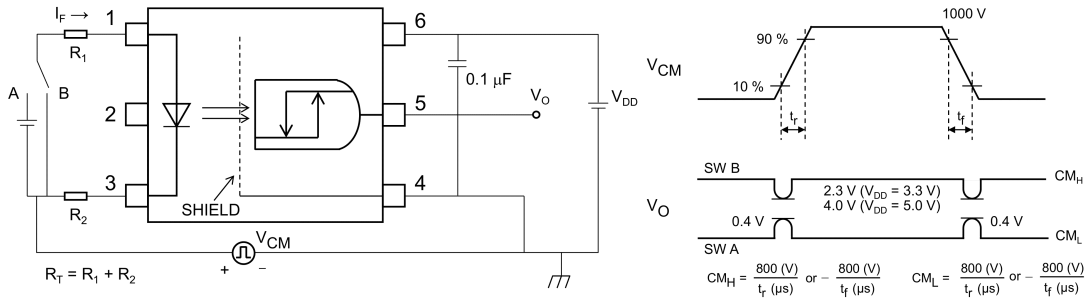
図 13.1.7 コモンモード過渡耐性測定回路, 波形
