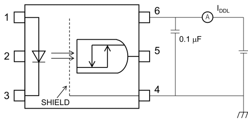
図 13.1.3 I_{DDL} 測定回路
