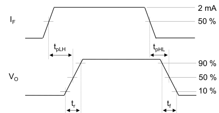
図 13.1.6 伝搬遅延時間測定回路, 波形
