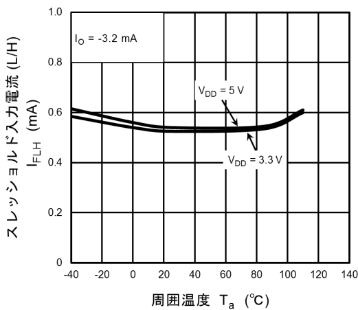
図 13.2.9 I_{FLH} - T_a
