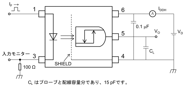
図 13.1.6 伝搬遅延時間測定回路, 波形
