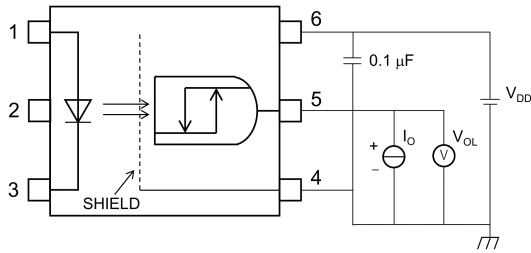
図 13.1.1 V_{OL} 測定回路
