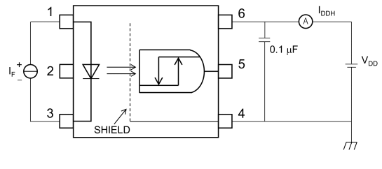
図 13.1.4 I_{DDH} 測定回路
