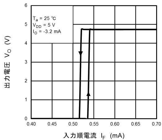
図 13.2.10 V_O - I_F
