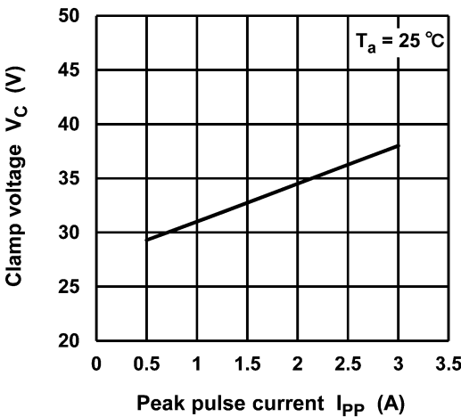
Fig. 10.1 V_C - I_{PP}
