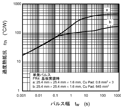
図 8.11 r_{th} - t_w
