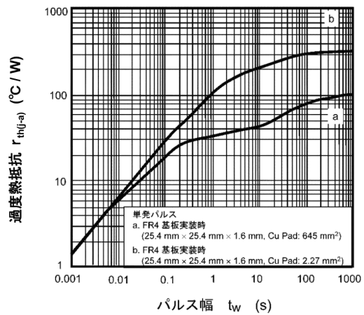
図 9.12 r_{th(j-a)} - t_w
