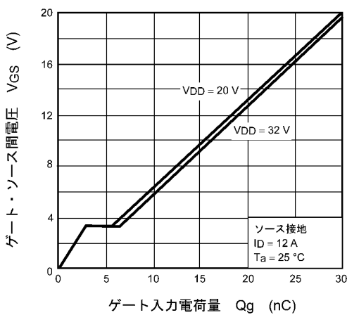
図 9.11 ダイナミック入力特性
