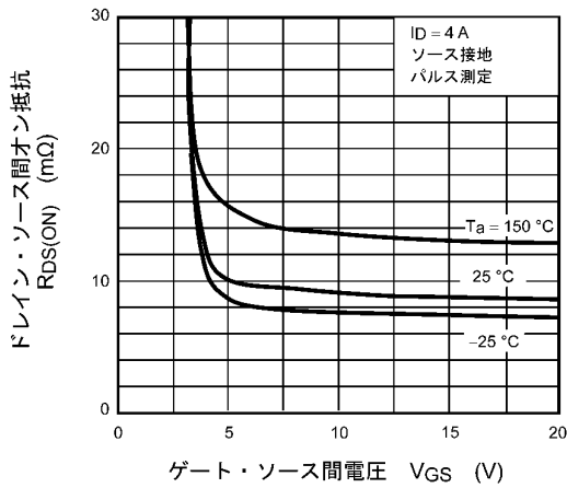
図 9.3 R_{DS(ON)} - V_{GS}
