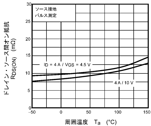
図 9.6 R_{DS(ON)} - T_a
