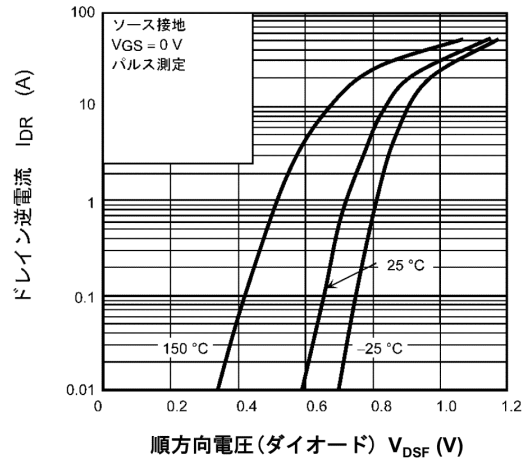
図 9.8 I_{DR} - V_{DSF}
