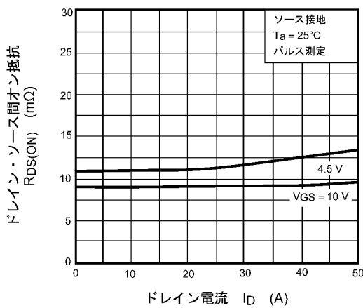
図 9.5 R_{DS(ON)} - I_D
