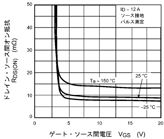
図 9.4 R_{DS(ON)} - V_{GS}
