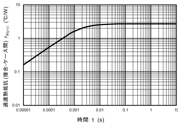
図 9.5 r_{th(j-c)} - t (最大値(保証値))
