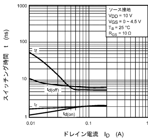
図 7.11 t - I_D
