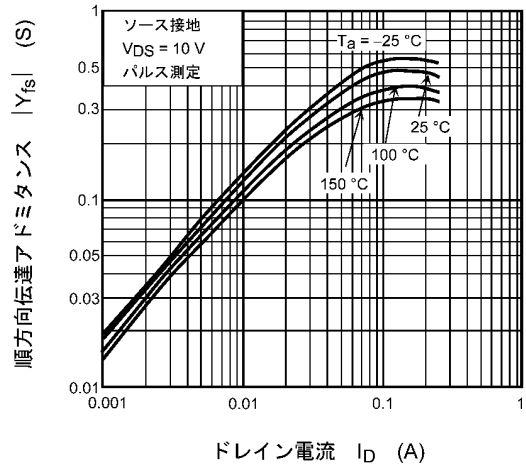
図 7.8 |Y_{fs}| - I_D
