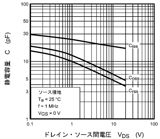
図 7.10 C - V_{DS}
