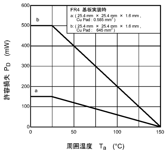
図 7.13 P_D - T_a
