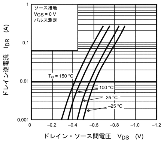
図 7.9 I_{DR} - V_{DS}
