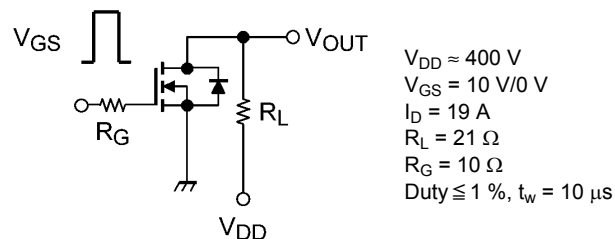
図 6.2.1 スwitching時間の測定回路
