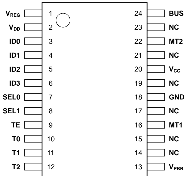
图 5.1 端子配置图
