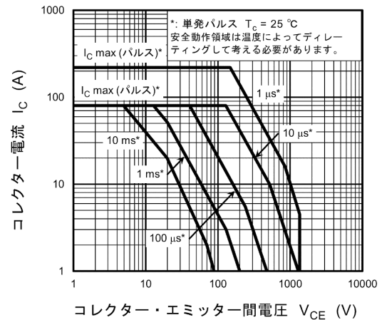
図 8.10 安全動作領域 (最大値 (保証値))
