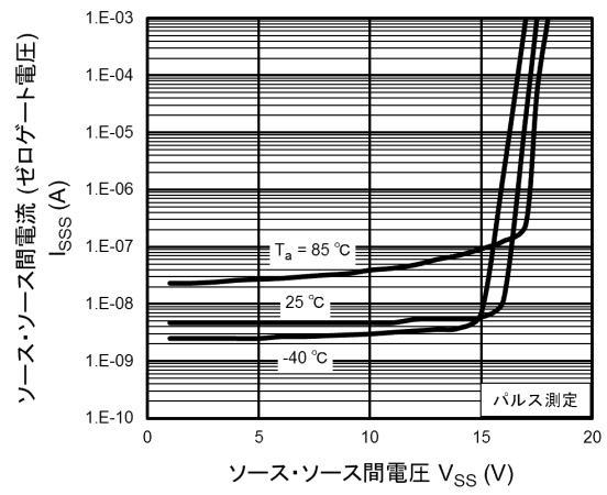
図 9.6 I_{CSS} - V_{SS}
