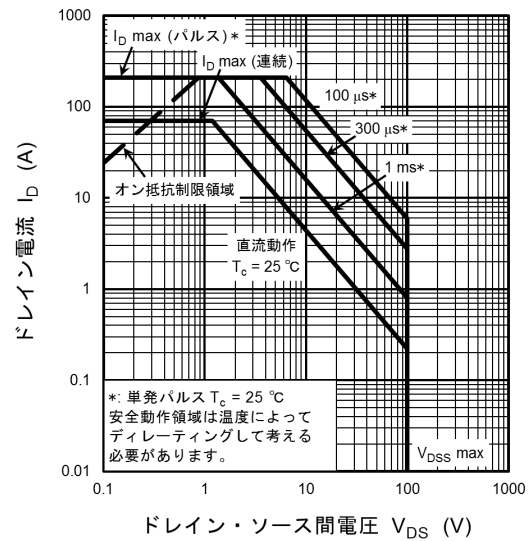
図 8.19 安全動作領域 (最大値 (保証値))
