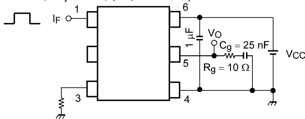
図 13.1.7 伝搬遅延時間測定回路, 波形
